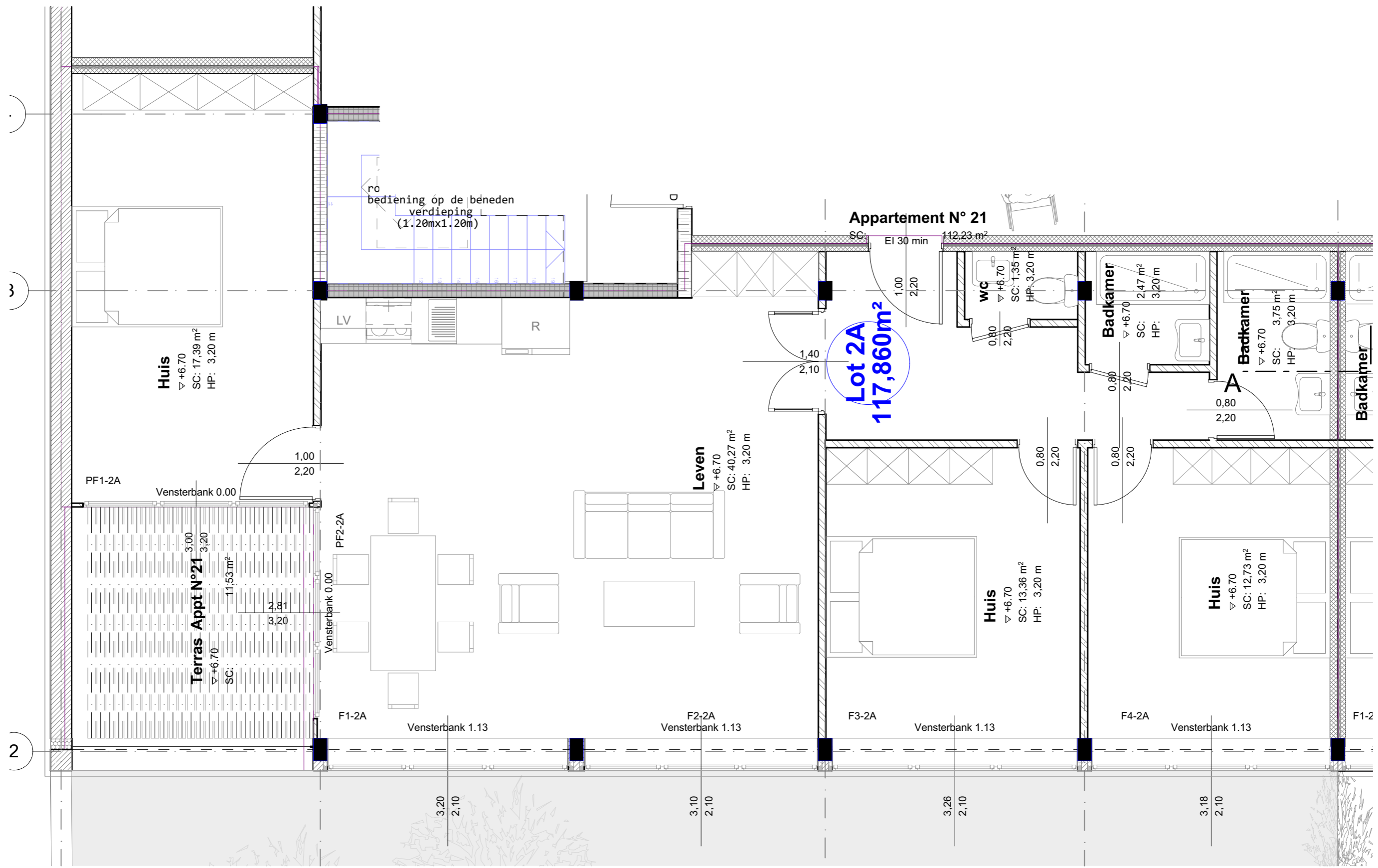
2. 2ème étage 1:50
